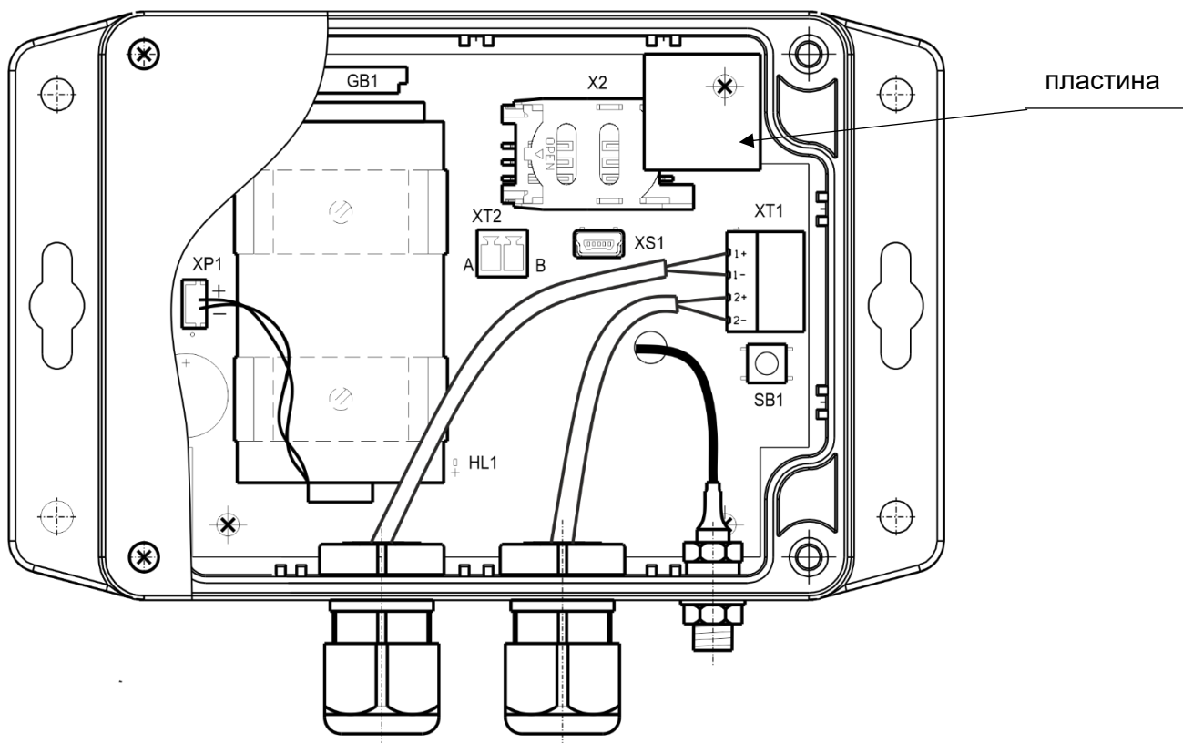
Рисунок 2 – Модуль SML-N2 со снятой крышкой
