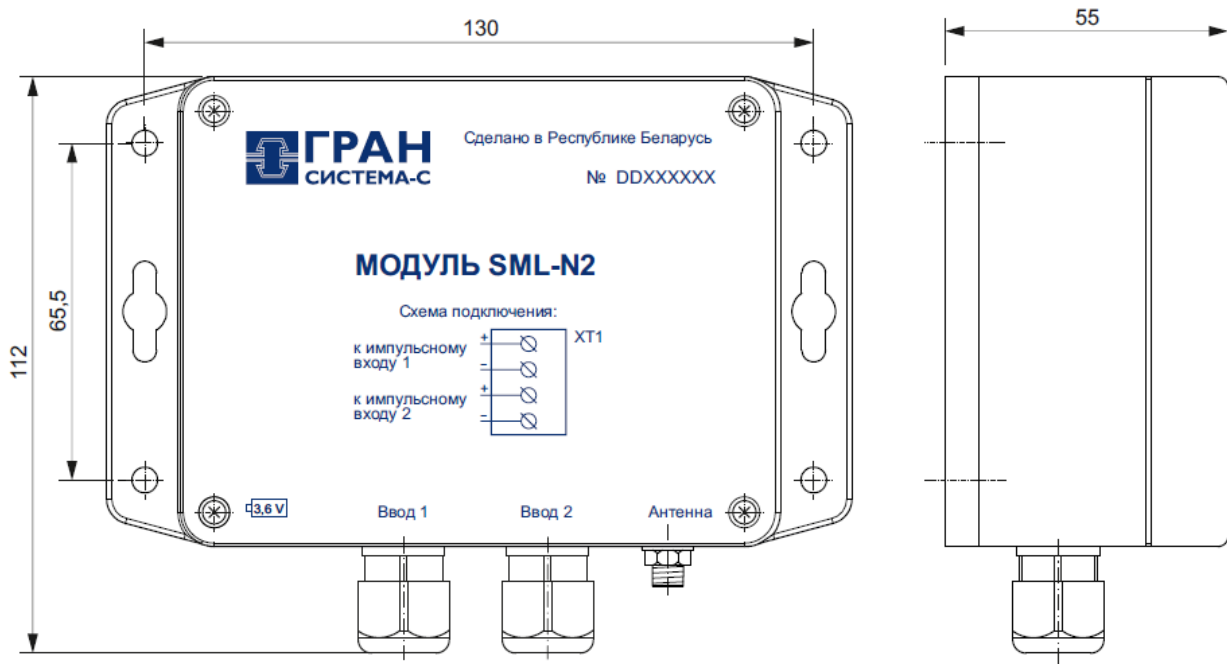
Рисунок А.1 – Габаритные и установочные размеры модулей SML-N2
